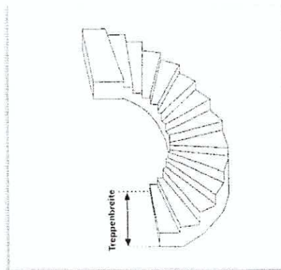
4 Wendeltreppe 180° gebogen
